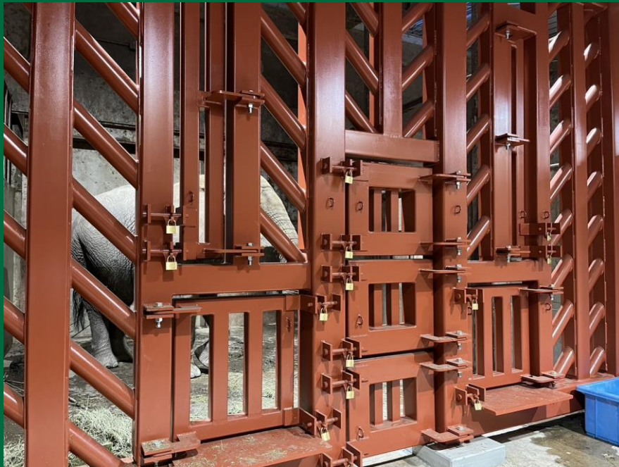
PCウォール全体図 (プロテクテッド・コンタクト・ウォール)
